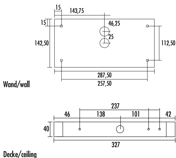
Bohrabstände SR / drilling distances SR
